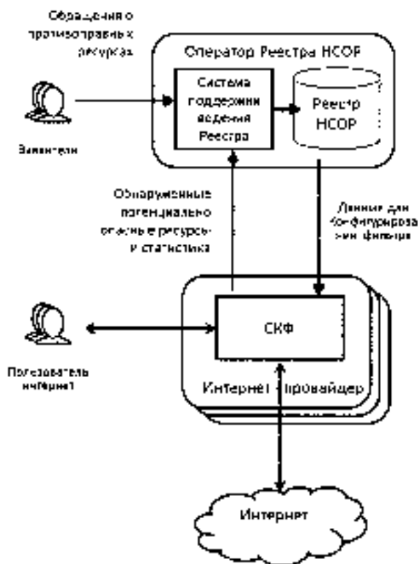
Рисунок 6. Принцип контроля доступа через Реестр NSOP
